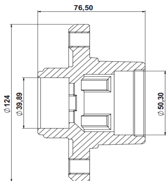
SEÇÃO A-A
