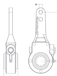
DESENHO TÉCNICO
