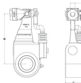
DESENHO TÉCNICO
